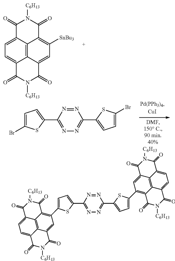
NDI-BTTZ-NDI
