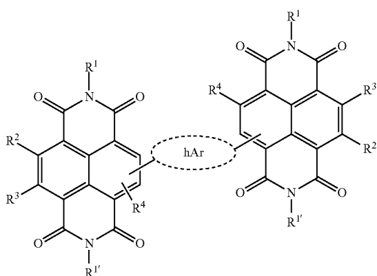
"NDI-hAr-NDI"
