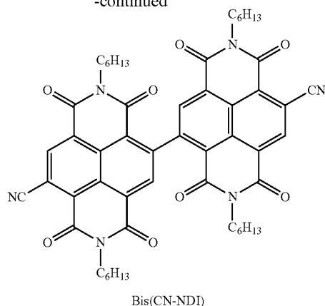
Bis(CN-NDI)
