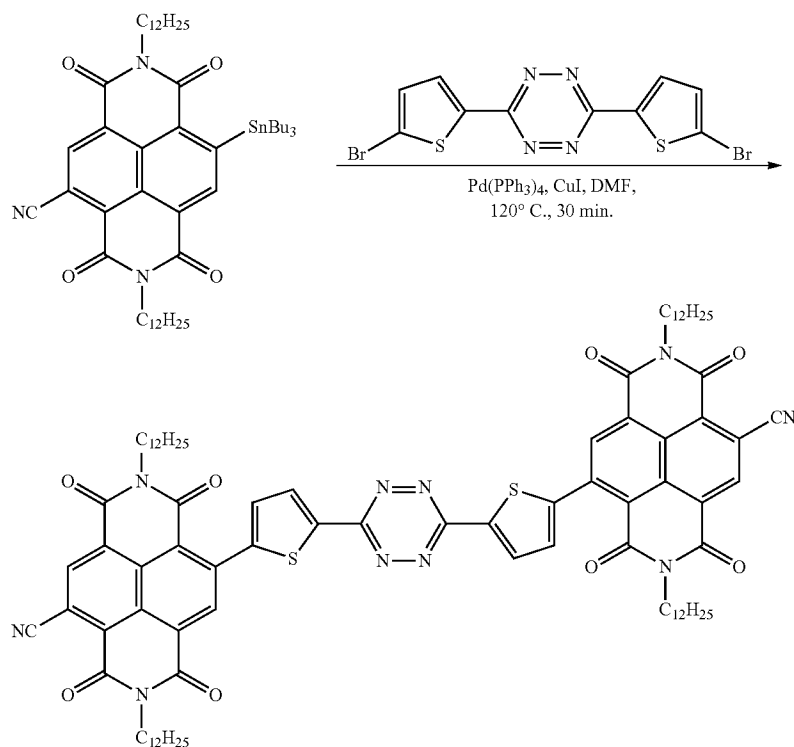
Bis(CN-NDI12)BTZ
