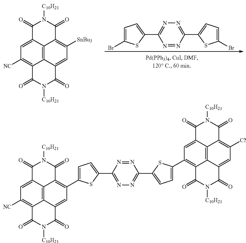
Bis(CN-NDI10)BTZ
