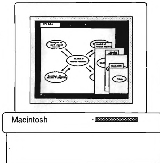
OFMdraw
