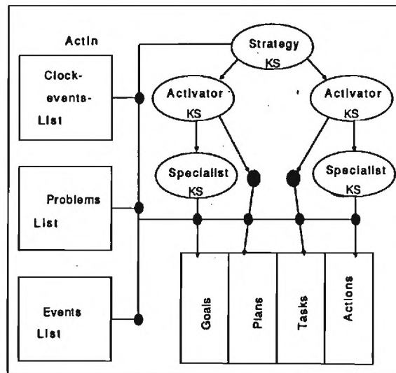
OFMspert
